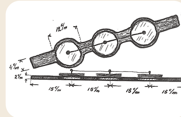
De bouwtekening van de matrimonial
